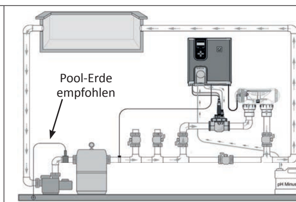
Installation als Bypass
