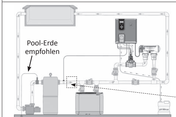
Installation mit einer Heizanlage
